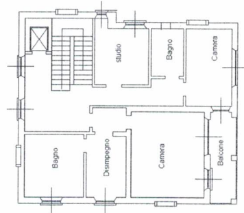
PIANO TERRENO H.3.15 M
